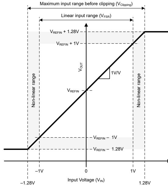
图 7-2. AMC0x30S-Q1 的输入到输出传递曲线
