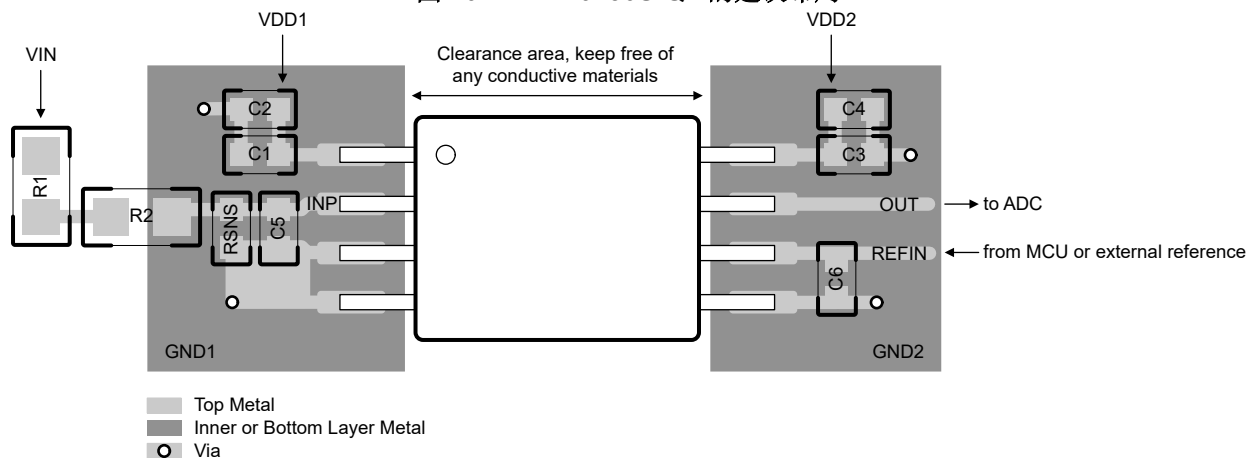
图 10-1. AMC0x30S-Q1 的建议布局
