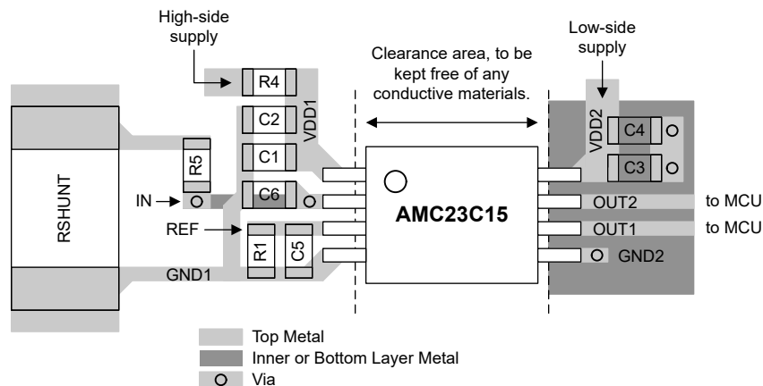
图 8-8. 建议布局 AMC23C15
