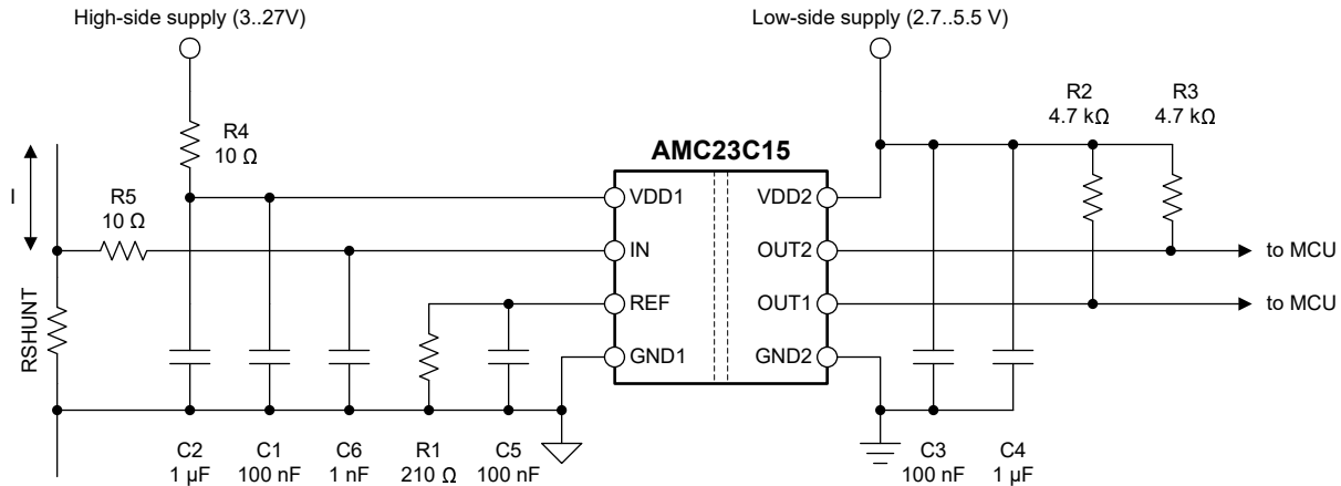
图 8-7. 去耦 AMC23C15
