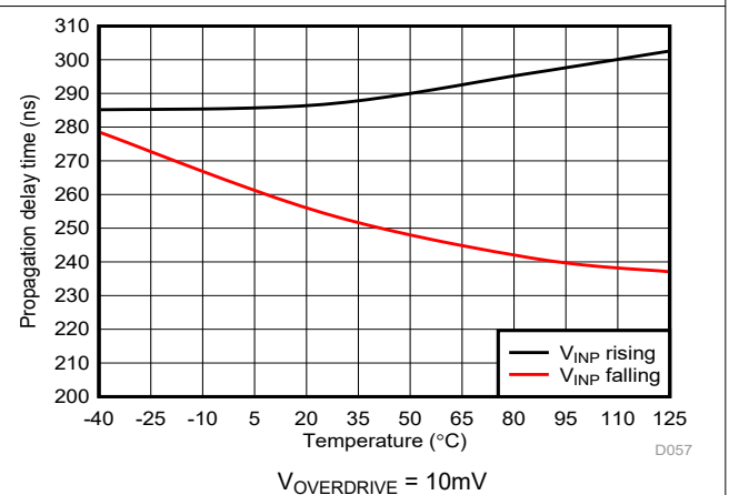
图 6-52. Cmp0 传播延迟与温度间的关系
