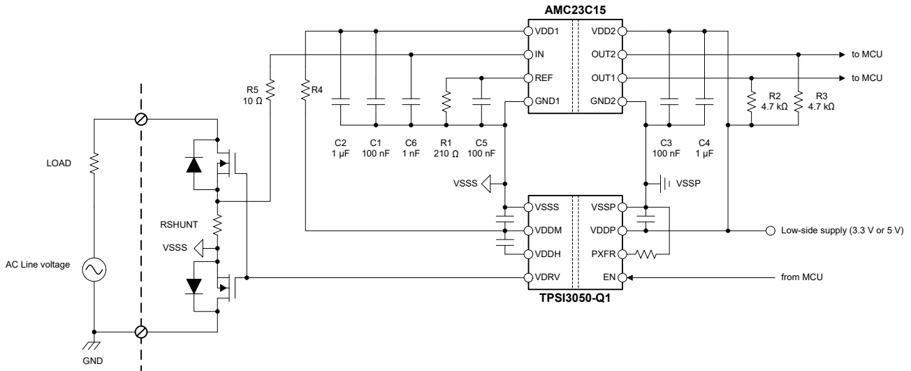
图 8-1. 使用 AMC23C15 进行过流和短路检测
