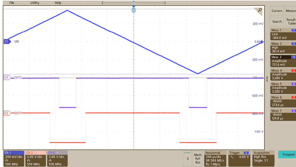
图 8-2. AMC23C15 对三角输入波形的输出响应
