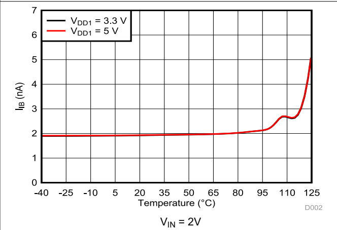
图 6-56. 输入偏置电流与温度间的关系
