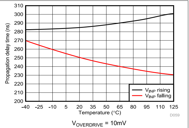
图 6-48. Cmp2 传播延迟与温度间的关系
