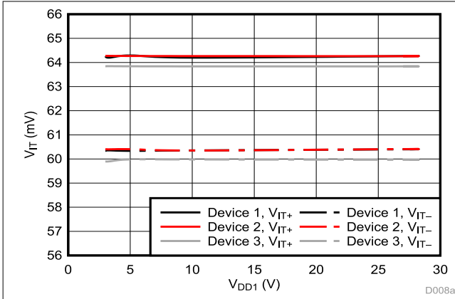
图 6-5. Cmp2 跳变阈值与电源电压间的关系
