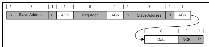
图 16. Single Read
