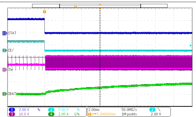
图 48. Charge Enable
