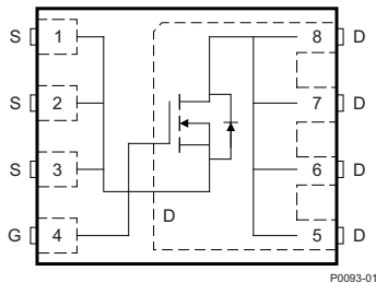
图 1. 顶视图
