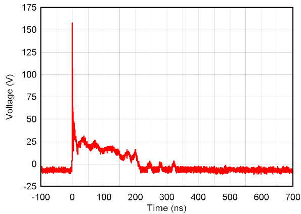
图 6-9. +8-kV Clamped IEC Waveform
