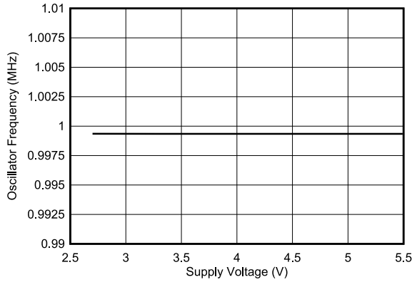
图 5-22. 内部时钟频率与电源间的关系
