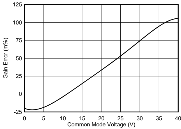
图 5-8. 电流增益误差与共模电压间的关系
