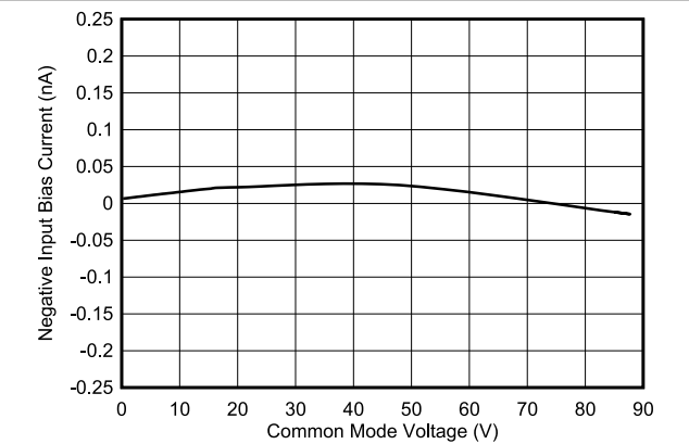
图 5-13. 输入偏置电流 ( I_{B+} 或 I_{B-} ) 与共模电压间的关系
