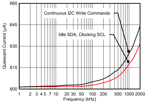
图 5-20. 工作 I_Q 与时钟频率间的关系
