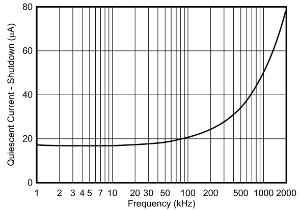
图 5-21. 关断 I_Q 与时钟频率间的关系
