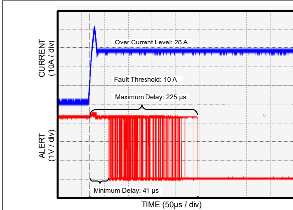
图 7-3. 警报响应时间 (采样值明显高于阈值)
