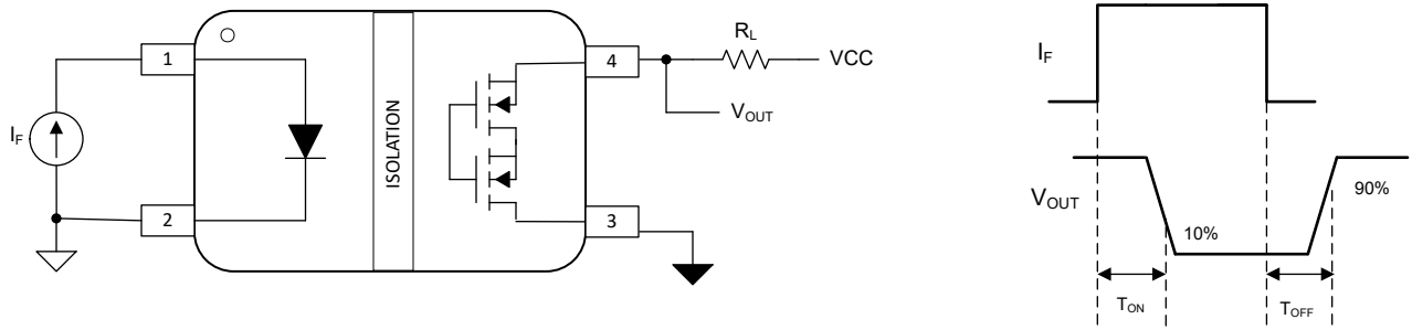
图 7-1. ISOM8610 导通和关断时间测试电路
