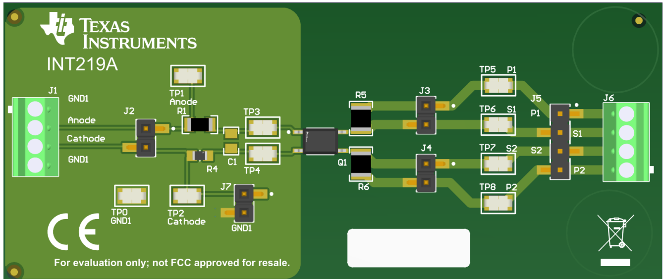
图 9-3. 采用 2 层电路板的 ISOM8610 布局示例
