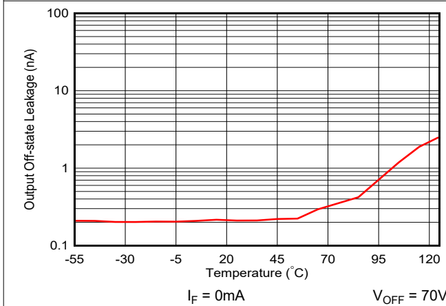
图 6-7. 关断状态漏电流与环境温度间的关系
