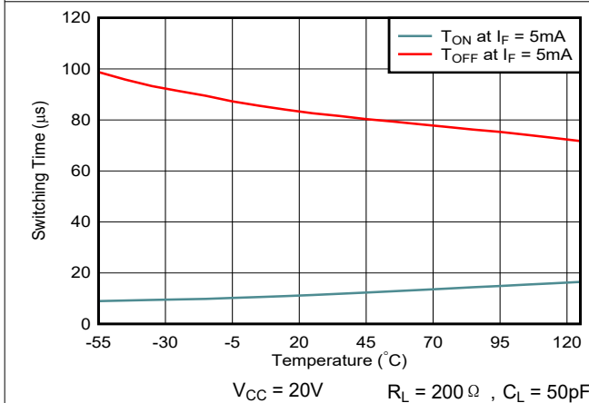
图 6-9. 导通和关断时间与环境温度间的关系
