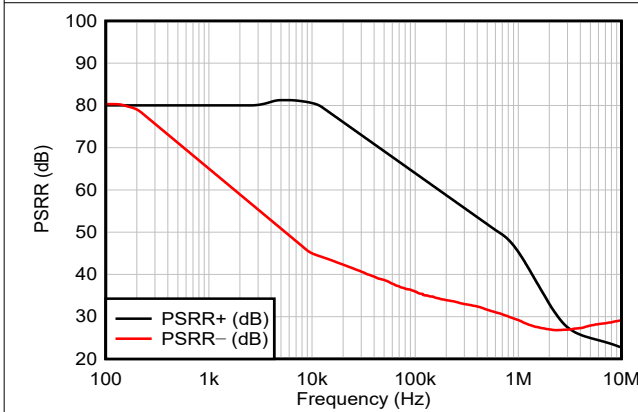
图 6-9. PSRR 与频率间的关系
