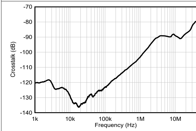
图 6-33. 通道隔离与频率间的关系
