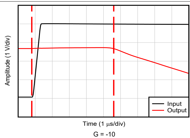
图 6-24. 过载恢复 (正轨)
