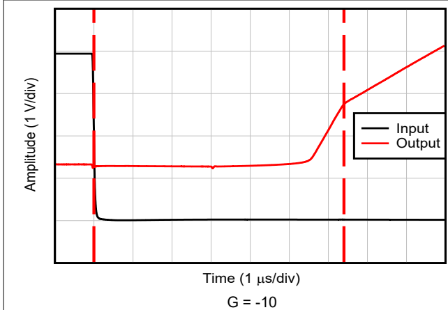
图 6-25. 过载恢复 (负轨)
