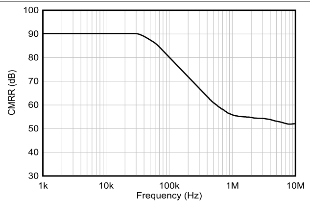
图 6-8. CMRR 与频率间的关系
