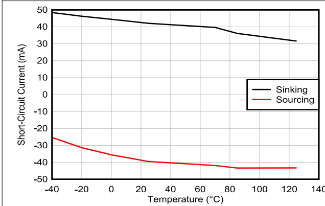
图 6-31. 短路电流与温度间的关系
