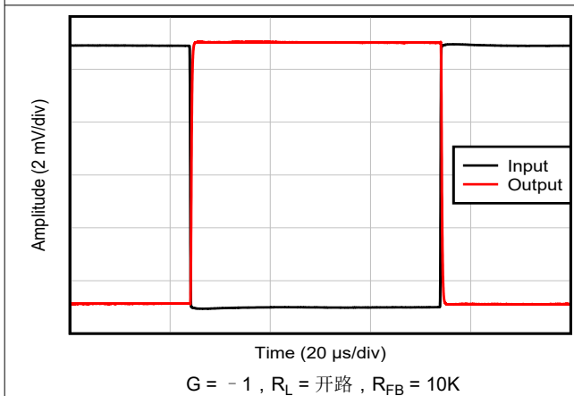
图 6-27. 小信号阶跃响应, G = -1
