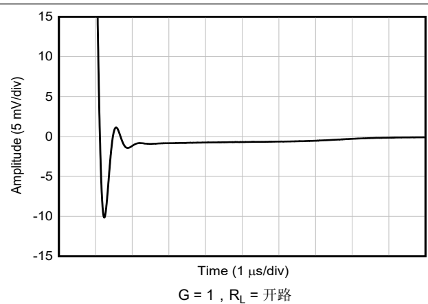
图 6-28. 大信号阶跃响应 (下降)
