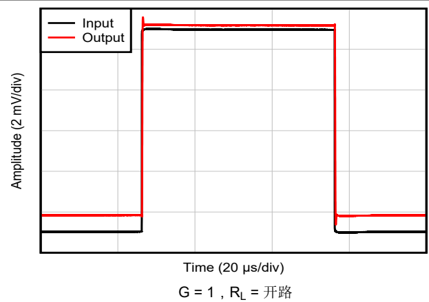
图 6-24. 过载恢复 (正轨)
