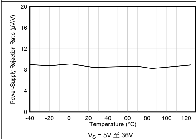
图 6-11. 电源抑制比与温度间的关系 (dB)
