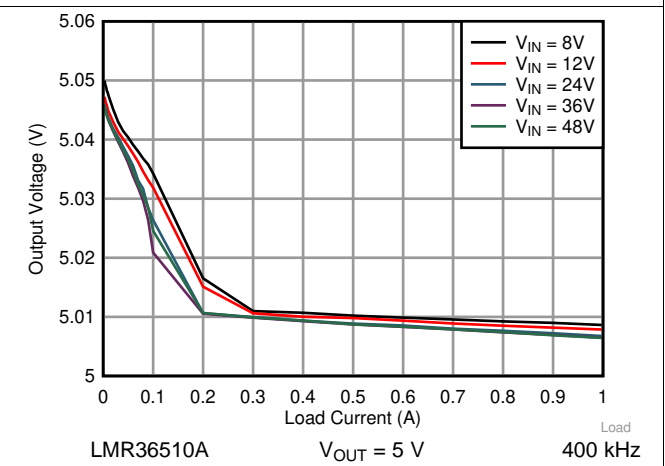
图 19. Load Regulation
