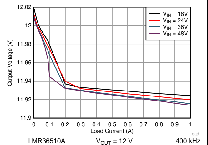
图 21. Load Regulation
