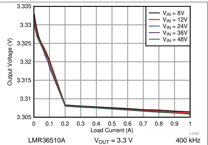
图 17. Load Regulation
