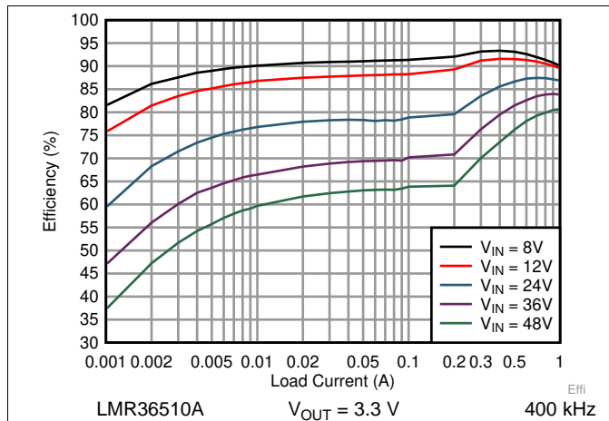
图 16. Efficiency
