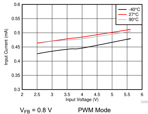
图 6-6. Non-Switching Input Current in PWM Mode
