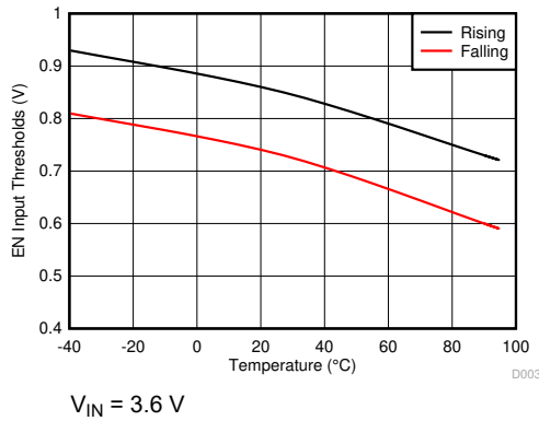
图 6-3. EN Input Thresholds
