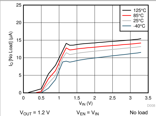
图 6-8. I_Q vs V_{IN}
