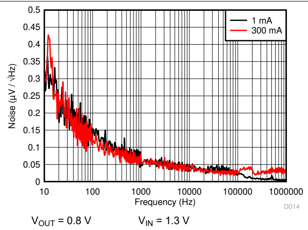
图 6-14. Noise Density
