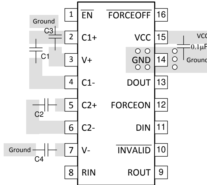
图 8-4. MAX3221E Layout Example
