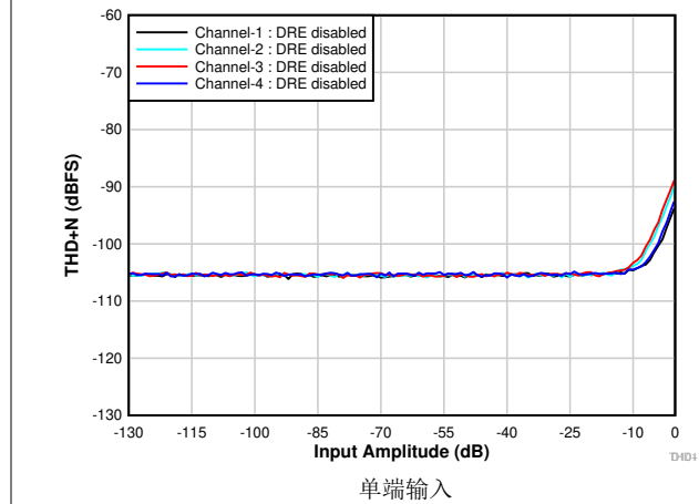
图 6-8. THD+N 与输入幅度间的关系 (DRE 已禁用)
