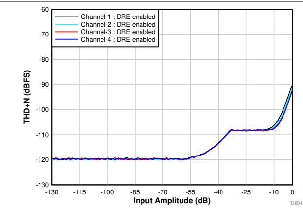
图 8-3. THD+N 与输入幅度间的关系 (DRE 已启用)
