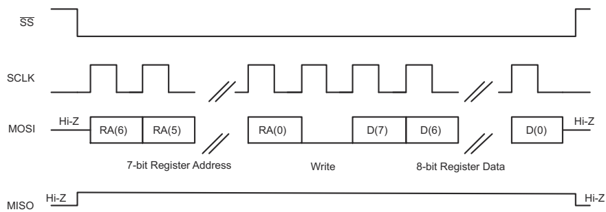
图 7-71. SPI 单字节写入传输
