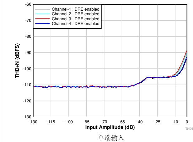
图 6-7. THD+N 与输入幅度间的关系 (DRE 已启用)
