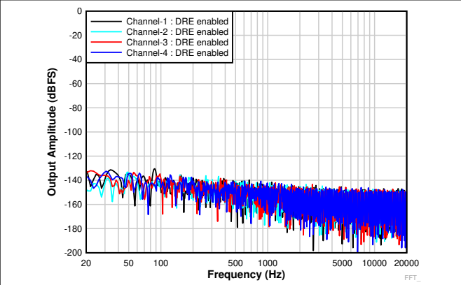
图 6-17. 空闲输入时的 FFT ( DRE 已启用 )
