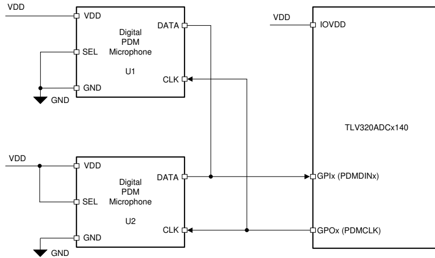
图 7-64. 数字 PDM 麦克风与以下器件的连接图：PCM5140-Q1
