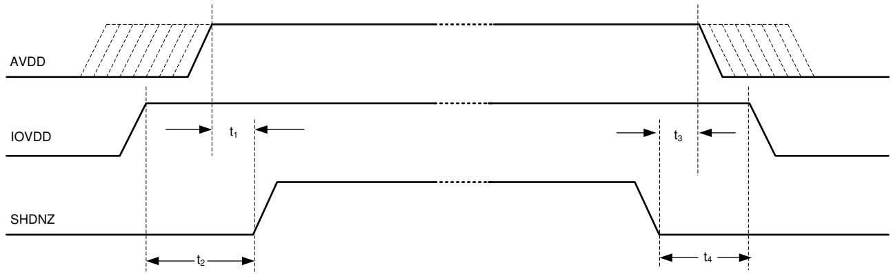
图 9-1. 电源时序要求时序图
