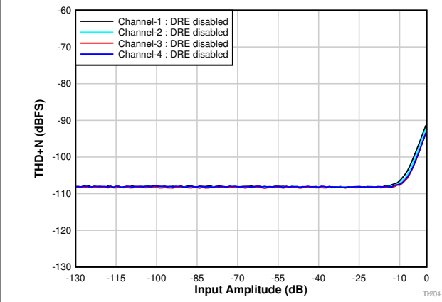
图 8-5. THD+N 与输入幅度间的关系 (DRE 已禁用)
