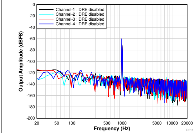
图 8-4. 具有 -60dB r 输入的 FFT (DRE 已禁用)
