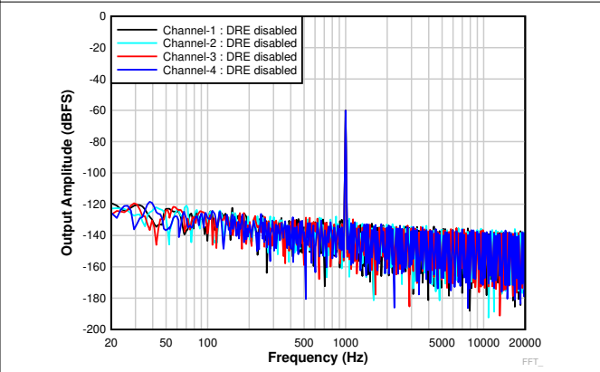
图 6-20. 具有 -60dBm 输入的 FFT ( DRE 已禁用 )
