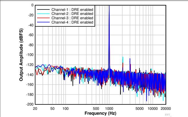
图 6-21. 输入为 -1dBm 时的 FFT ( DRE 已启用 )
