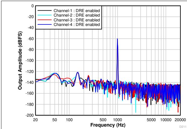
图 8-2. 具有 -60dB r 输入的 FFT (DRE 已启用)
