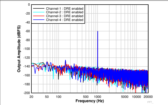
图 6-19. 输入为 -60dBm 时的 FFT ( DRE 已启用 )
