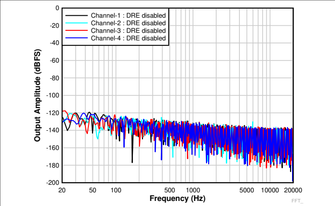
图 6-18. 空闲输入时的 FFT ( DRE 已禁用 )
