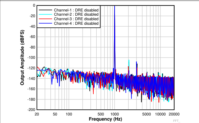
图 6-22. 具有 -1dBm 输入的 FFT ( DRE 已禁用 )
