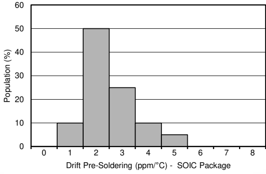
图 7-4. 焊接前漂移分配, SOIC 封装
