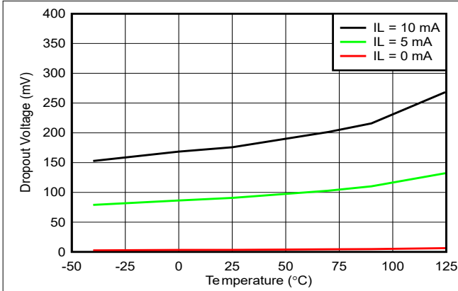
图 6-43. 压降电压与温度间的关系
