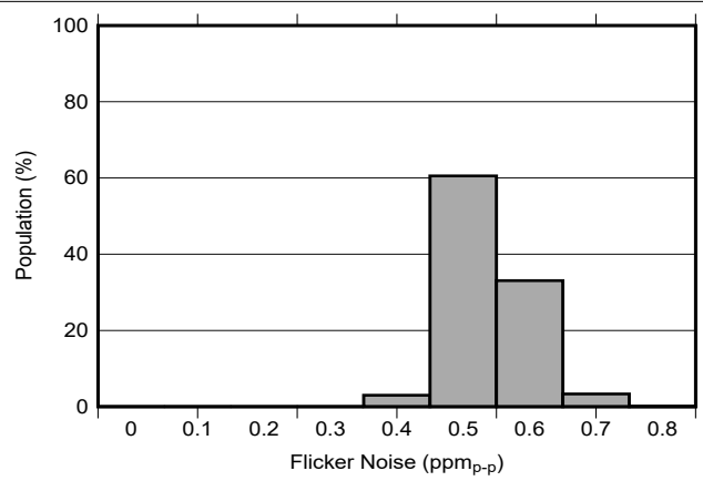
图 6-44. 0.1Hz 至 10Hz 电压噪声分布 ( C_{NR} = \text{开路} )
