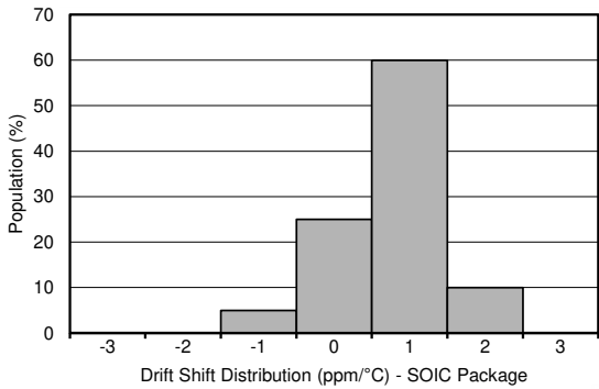
图 7-8. 漂移移位分配, SOIC 封装
