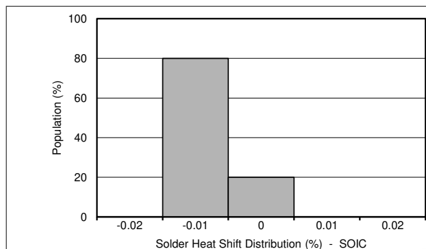
图 7-2. 焊接热移位分配 (%), SOIC 封装
