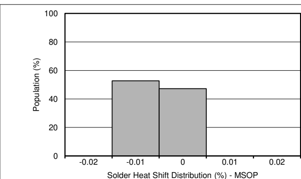
图 7-3. 焊接热移位分配 (%), VSSOP 封装
