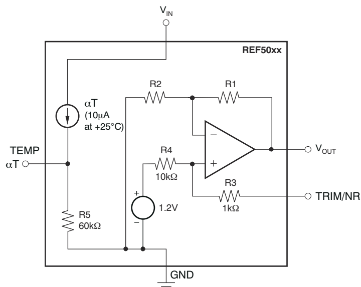
图 8-1. REF50xxI、REF50xxAI 方框图
