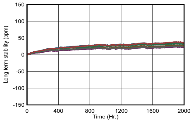
图 6-47. 长期稳定性 (前 2000 小时)
