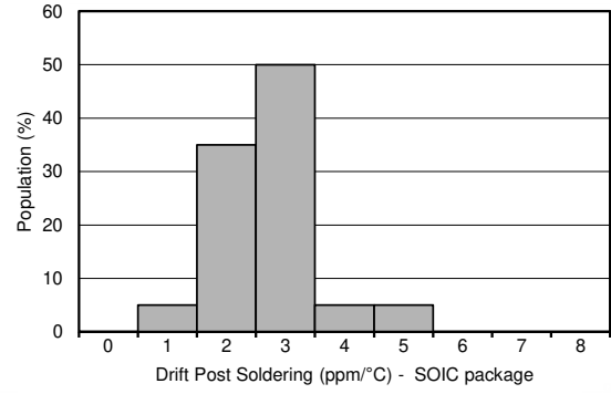
图 7-5. 焊接后漂移分配, SOIC 封装
