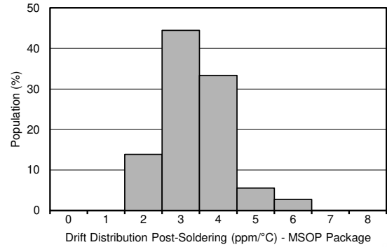
图 7-7. 焊接后漂移分配, VSSOP 封装
