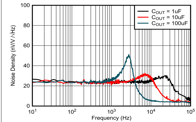
图 6-45. 噪声性能 10Hz 至 100kHz ( C_{NR} = \text{开路} )
