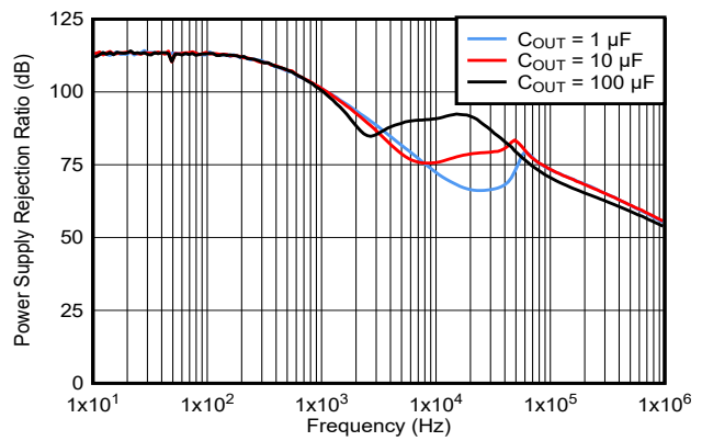
图 6-46. 电源抑制比与频率间的关系
