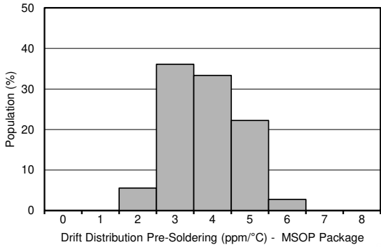
图 7-6. 焊接前漂移分配, VSSOP 封装
