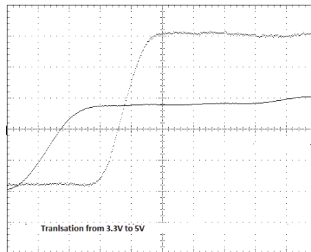
图 8-2. 升压转换
