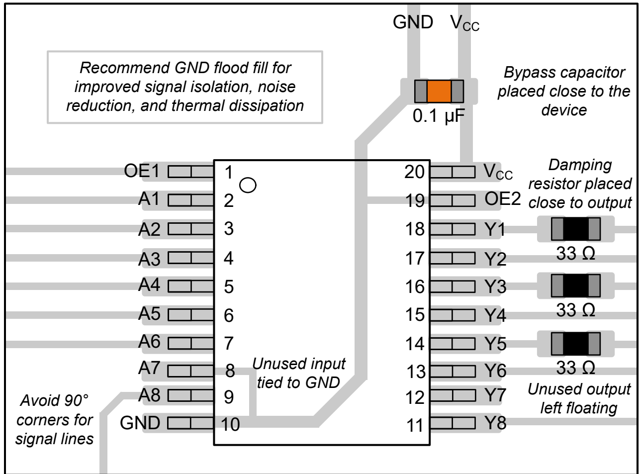
图 8-3. SN54SC8T541-SEP 的示例布局
