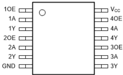
图 5-1. PW 封装，14 引脚（顶视图）
