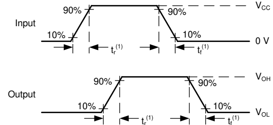
图 7-4. 电压波形，输入和输出转换时间
