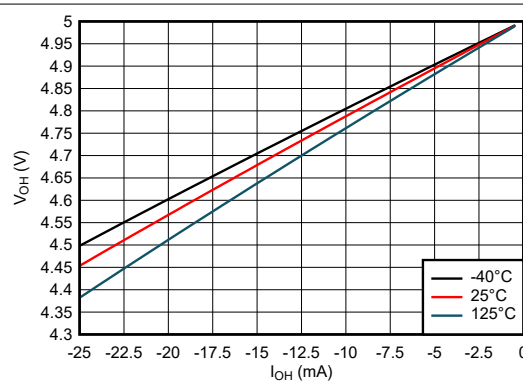
图 5-2. 高电平状态下输出电压与电流间的关系 (5V 电源)
