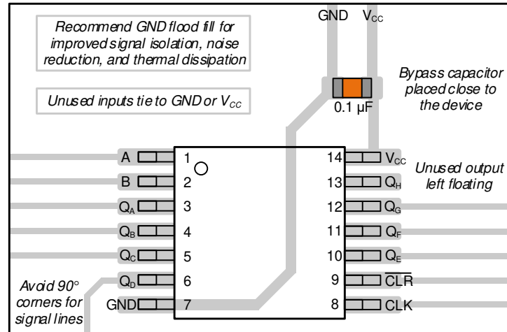
图 8-3. SN74AHC164 的示例布局
