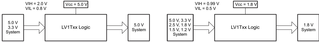
图 7-2. LV1Txx 升压和降压转换示例
