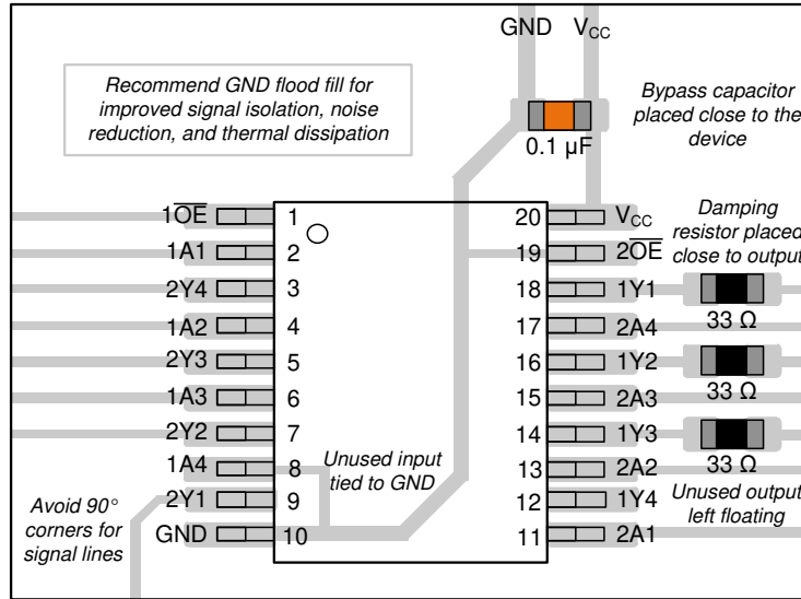
图 10-3. SN74LV8T244-Q1 采用 TSSOP 封装的示例布局
