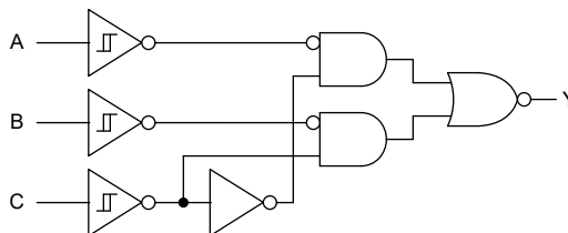
功能图
