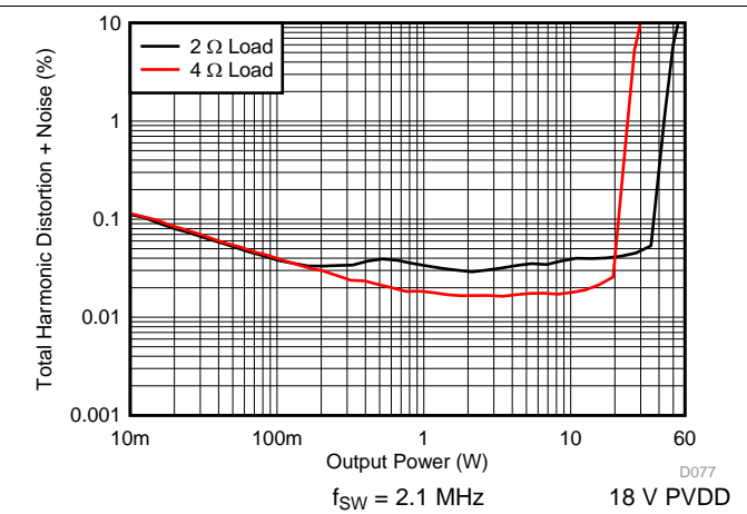
图 26. PBTL THD+N vs Power
