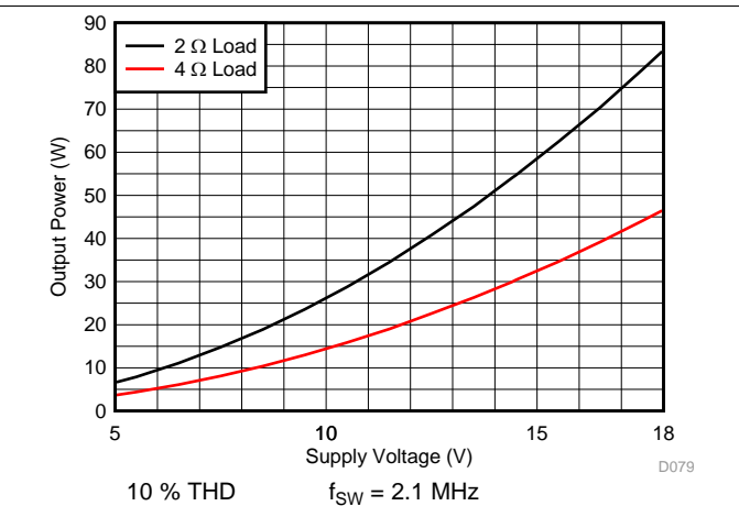
图 28. PBTL Output Power vs Voltage
