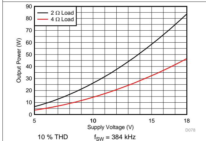
图 27. PBTL Output Power vs Voltage
