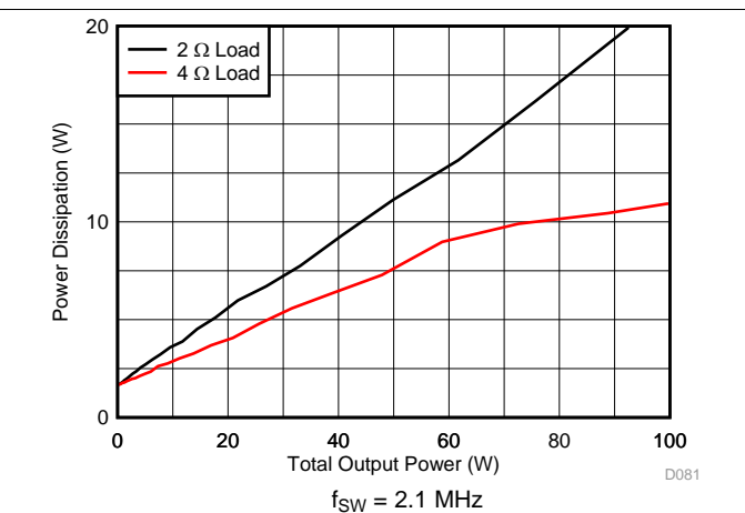
图 30. Power Dissipation vs Total Output Power
