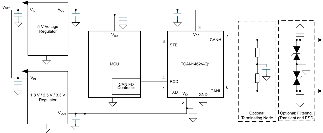
图 9-6. 使用 1.8V、2.5V、3.3V IO 连接的典型收发器应用
