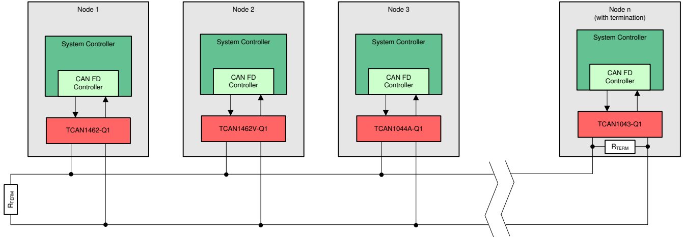
图 9-3. 典型 CAN 总线
