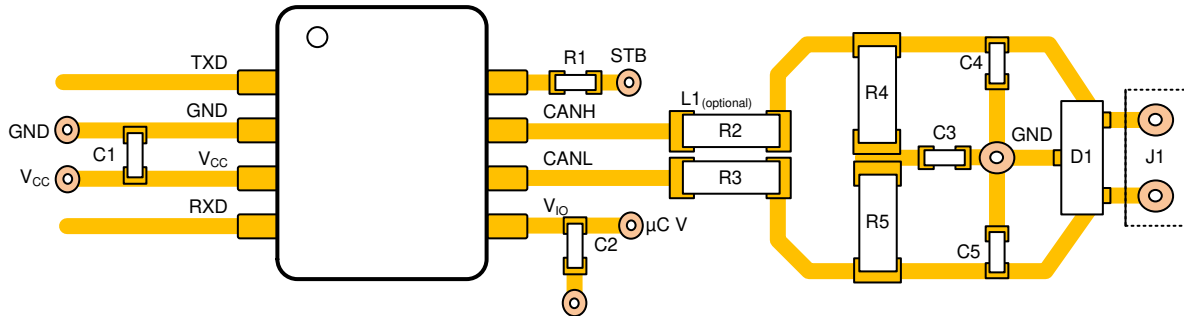
图 9-7. 布局示例
