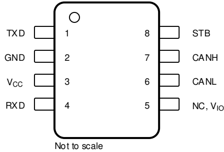
图 5-1. SOIC (D) 和 SOT-23 (DDF) 封装, 8 引脚 (顶视图)
