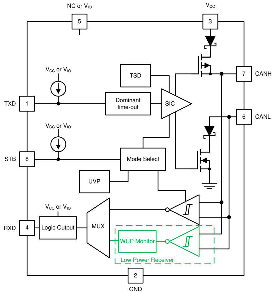
图 8-3. 方框图
