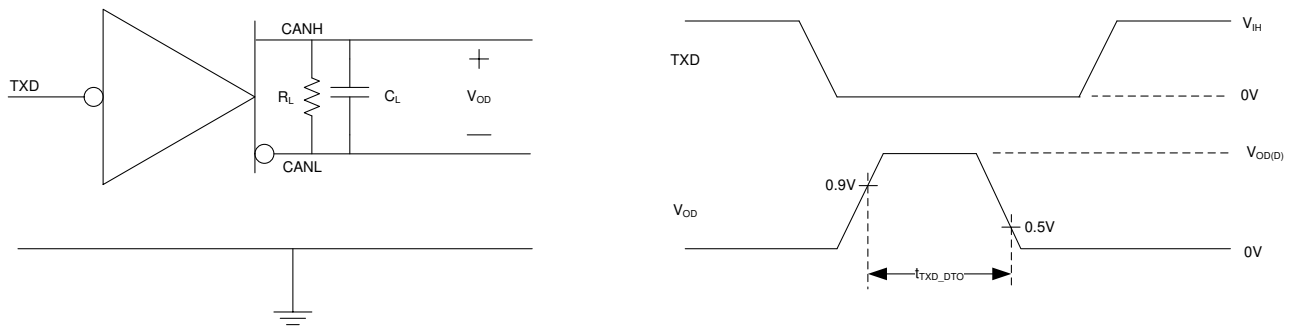
图 7-6. TXD 显性超时测试电路与测量
