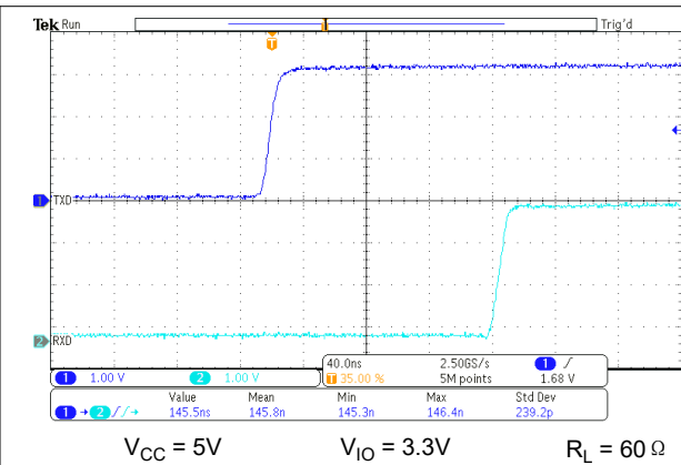
图 9-5. t_{PROP(LOOP2)}
