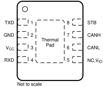
图 5-2. VSON (DRB) 封装, 8 引脚 (顶视图)
