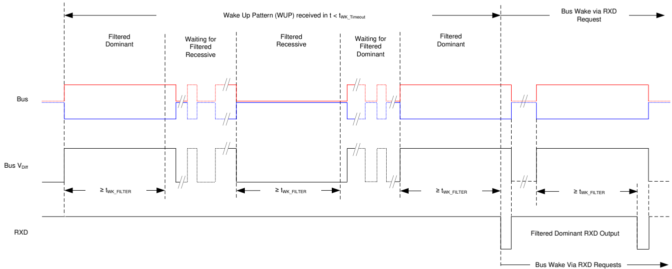
图 8-7. 具有 t WK_TIMEOUT 的唤醒模式 (WUP)
