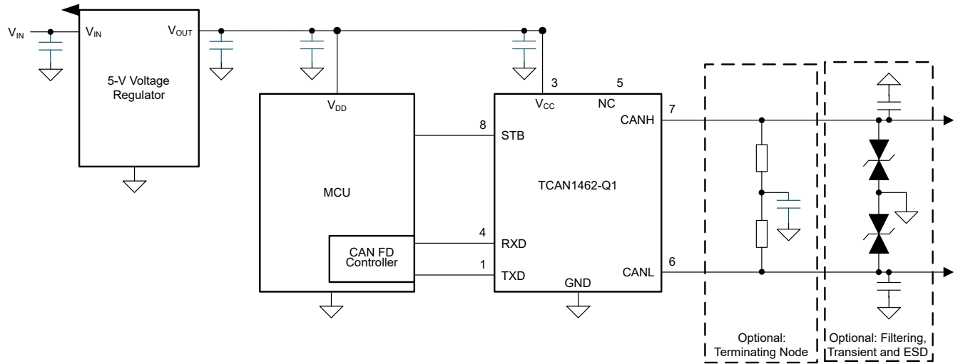
图 9-1. 使用 5V I/O 连接的收发器应用
