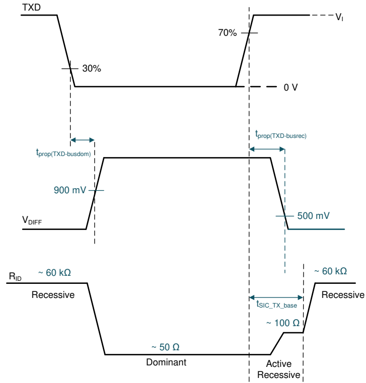
图 8-2. 基于 TX 的 SIC
