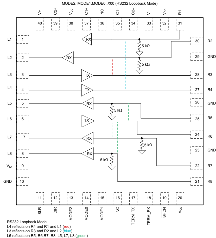
图 7-2. RS-232 Loopback Mode
