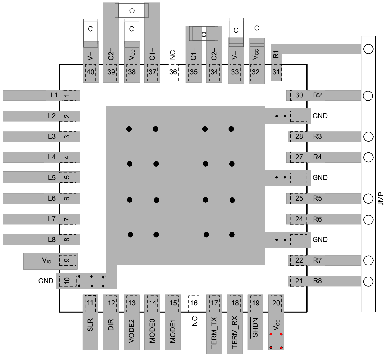
图 8-14. Layout Example
