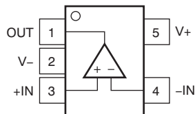
TLV171: DBV 封装 5 引脚 SOT-23 俯视图
