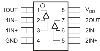
TLV272: D、DGK 和 P 封装 8 引脚 SOIC、VSSOP 和 PDIP 俯视图
