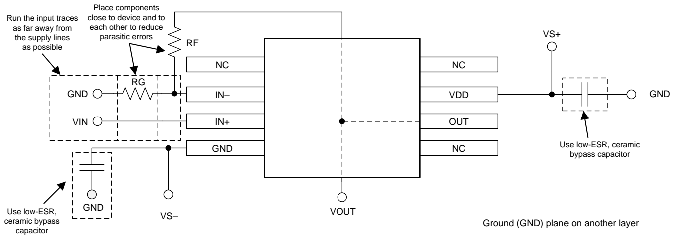
图 31. TLV27x 布局示例
