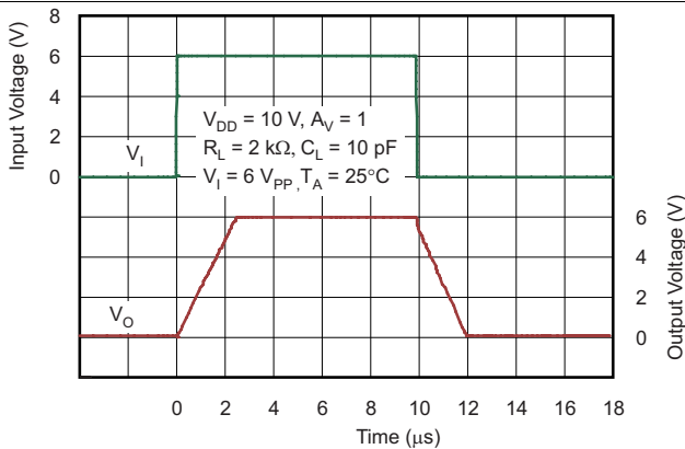
图 19. 电压跟随器大信号脉冲响应
