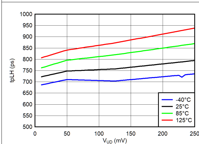
图 6-23. T_{PLH} vs Input Underdrive @ V_{CC} = 3.3\text{ V}
