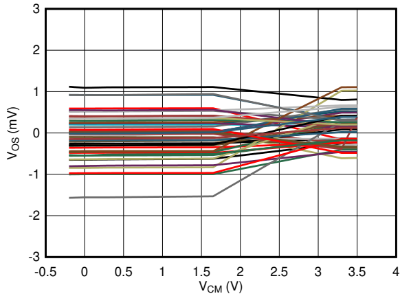
图 6-3. V_{OS} vs V_{CM} @ V_{CC} = 3.3\text{ V} - 50 Devices
