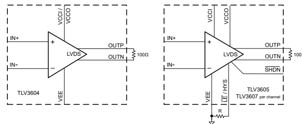
功能方框图
