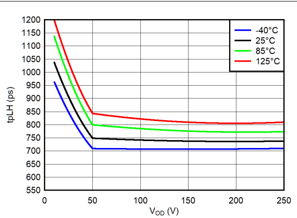
图 6-20. T_{PLH} vs Input Overdrive @ V_{CC} = 3.3\text{ V}
