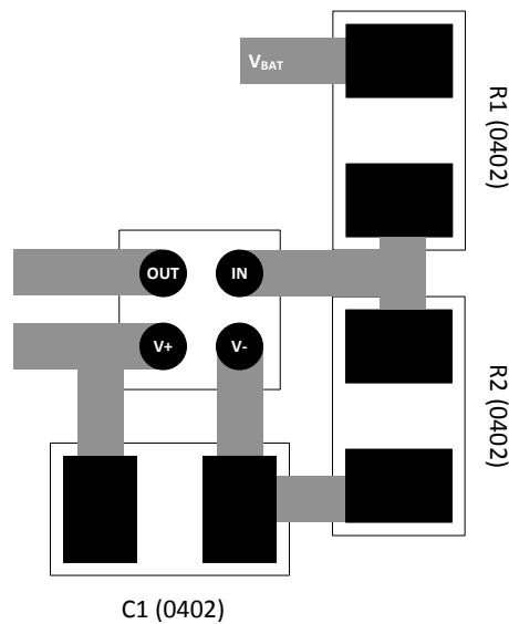
图 11-1. Layout Example
