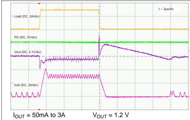
图 19. Load Transient
