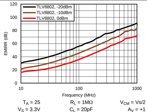
Figure 36. EMIRR 性能
