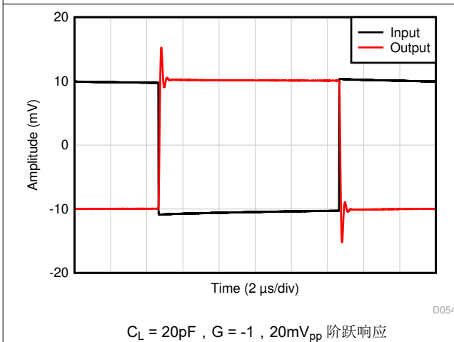
图 5-35. 小信号阶跃响应
