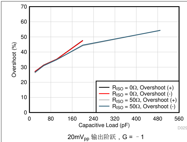
图 5-31. 小信号过冲与容性负载间的关系
