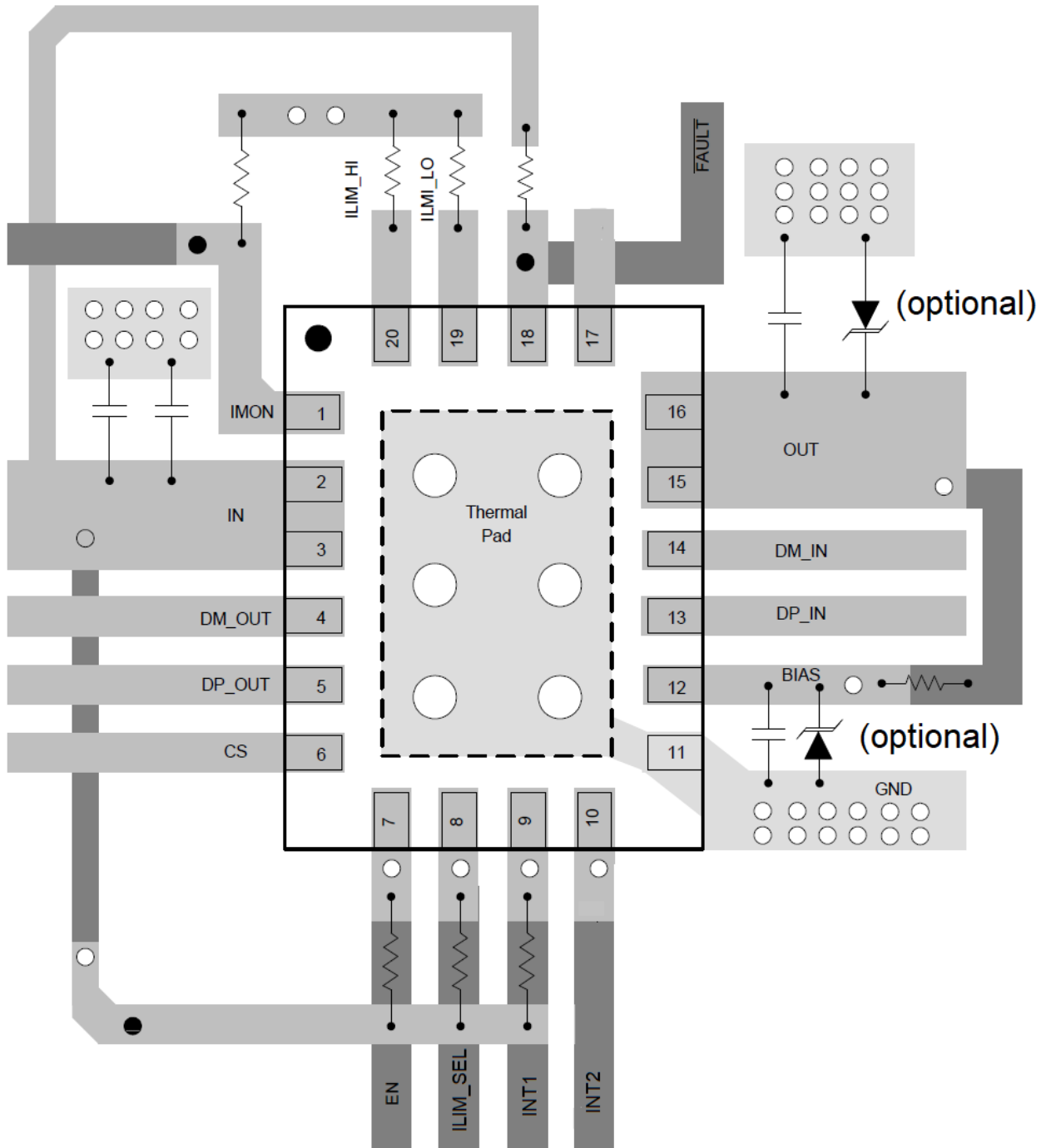
图 9-11. TPD3S713x-Q1 Layout Diagram
