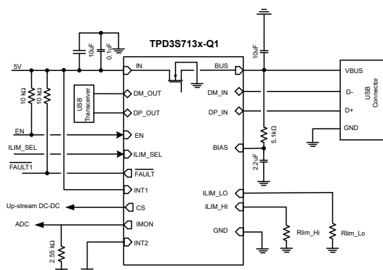
原理图
