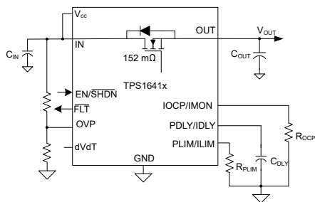
简化原理图
