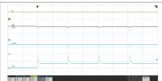
图 9-5. Transient Overload
