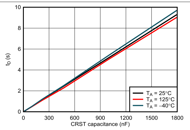
图 6-9. t_d 与电容间的关系
