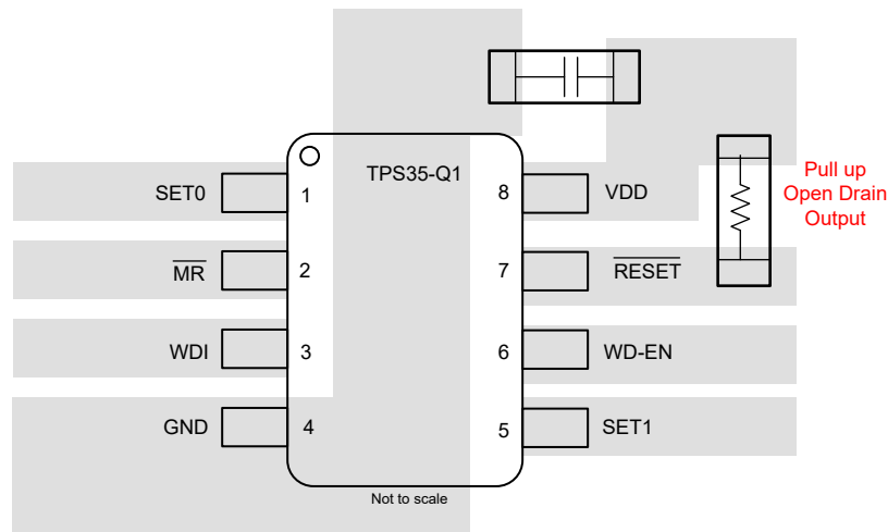
图 8-5. 引脚排列 C 的典型布局 - TPS35-Q1
