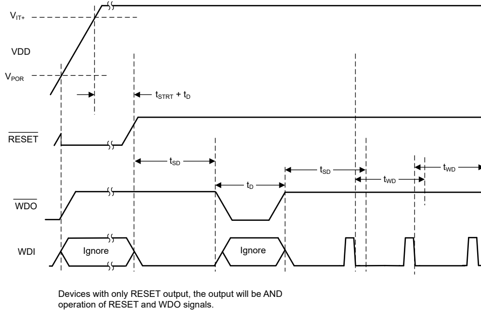
图 7-8. t_{SD} 帧行为
