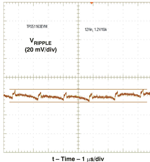
图 9-5. Output Ripple
