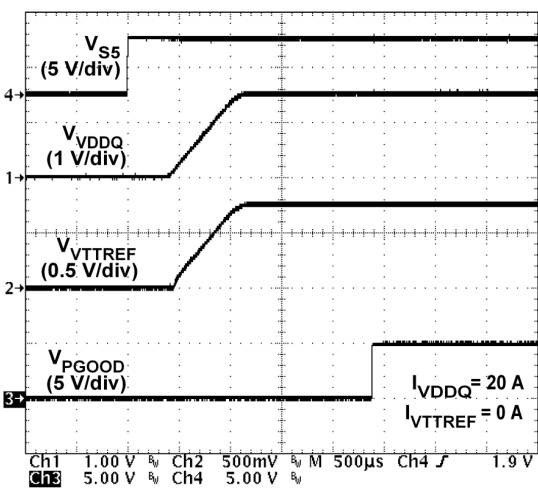
图 7-24. 1.5-V Startup Waveforms
