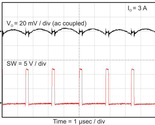
图 8-25. Tps563200 Output Voltage Ripple
