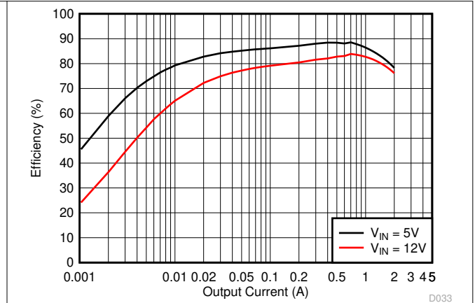
图 8-3. Tps562200 Light Load Efficiency
