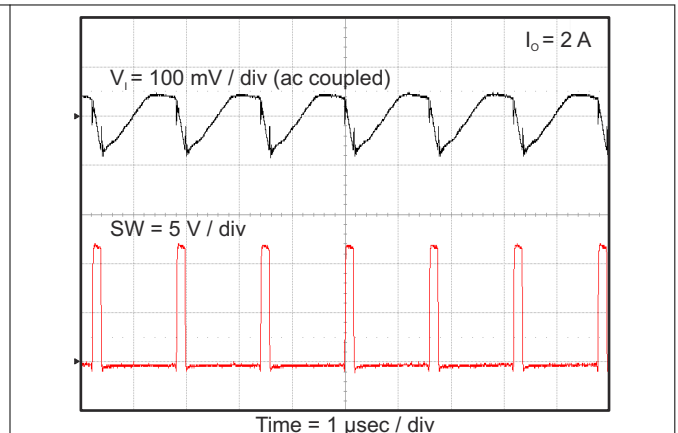
图 8-7. Tps562200 Input Voltage Ripple
