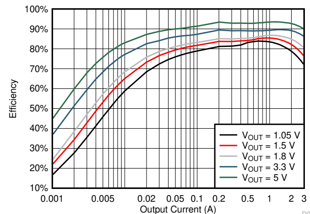
TPS563201 效率
