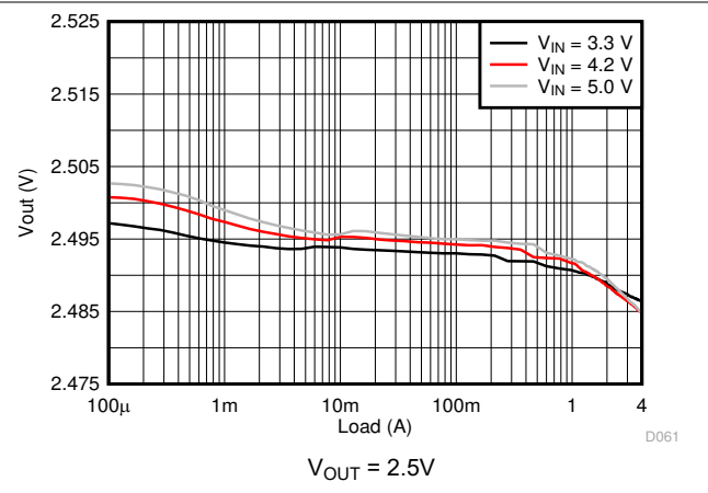
图 8-16. Load Regulation
