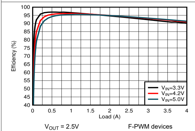
图 8-17. PWM Efficiency
