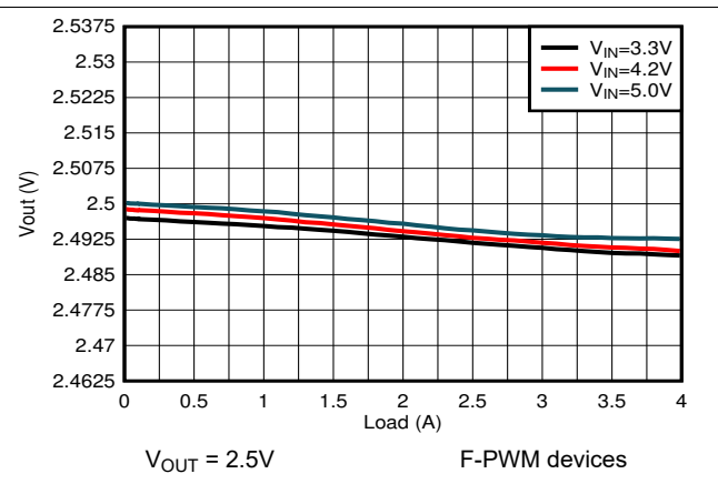
图 8-18. Load Regulation
