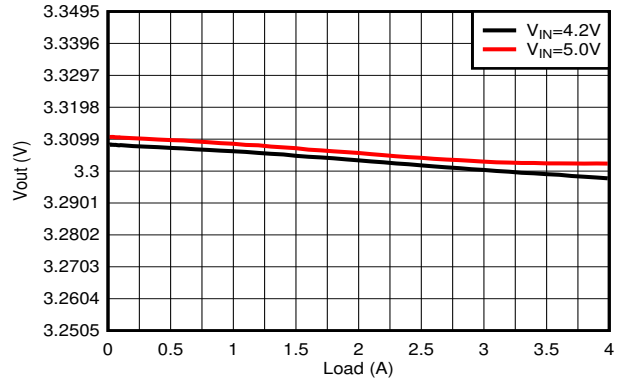
图 8-22. Load Regulation
