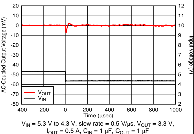
图 30. Line Transient
