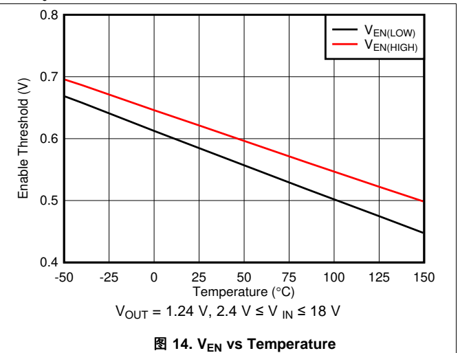
图 14. V_{EN} vs Temperature
