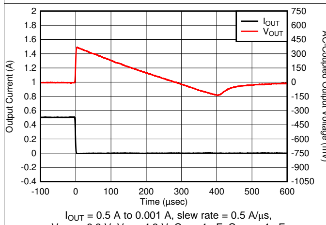
图 29. Load Transient
