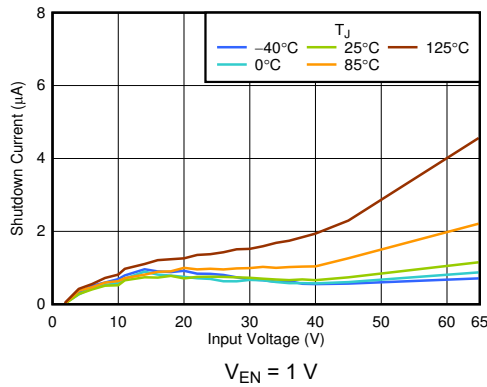
图 6-9. I_{SHUTDOWN} vs V_{IN}
