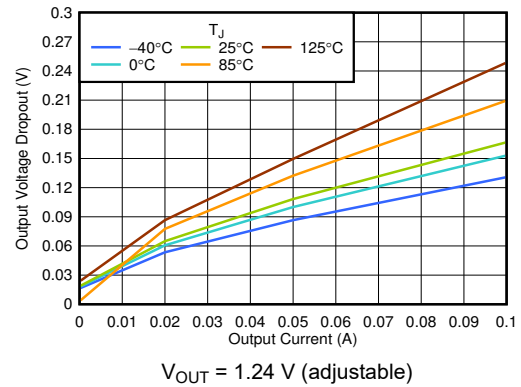
图 6-10. V_{DO(OUT)} vs I_{OUT}
