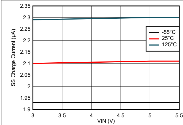
图 6-9. SS Charge Current Variation
