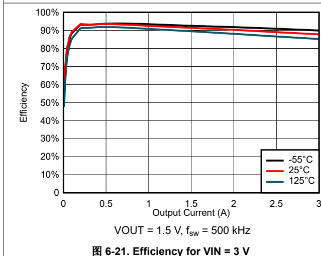
图 6-21. Efficiency for V_{IN} = 3\text{ V}
