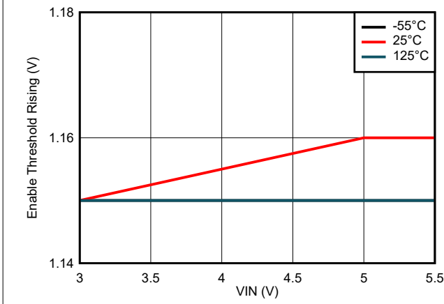
图 6-7. Enable Threshold Rising Variation
