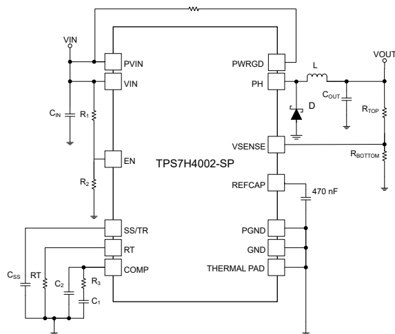
功能图
