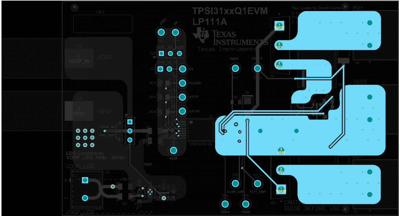
图 9-7. 信号层 2
