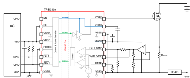
TPSI3100-Q1 简化原理图
