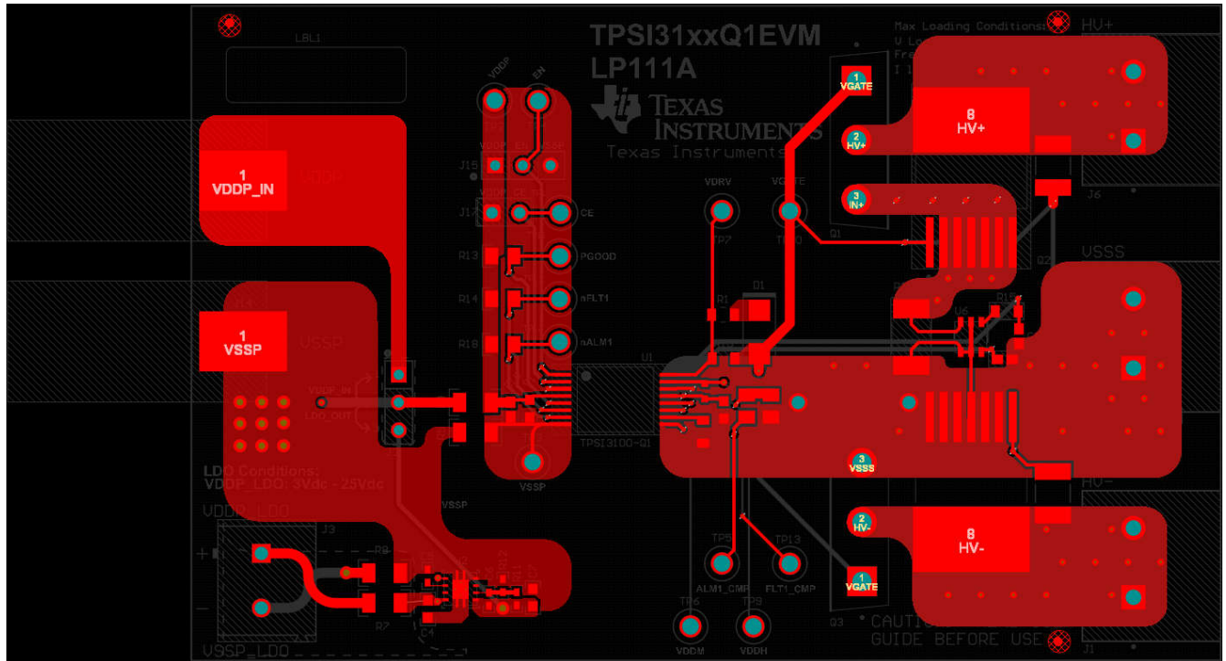
图 9-4. 顶层
