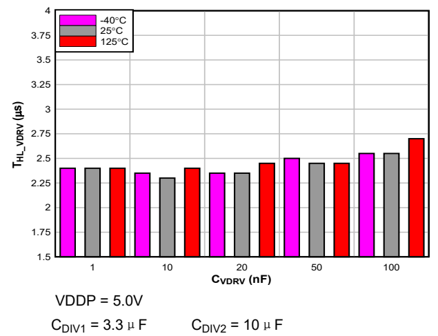
图 6-6. t HL_VDRV 与 C VDRV
