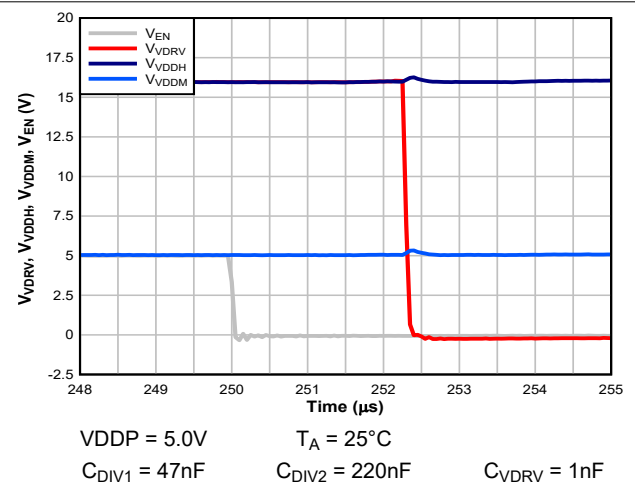
图 6-4. t HL_VDRV
