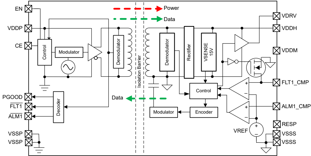
图 8-4. TPSI313x-Q1
