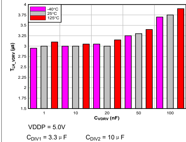
图 6-5. t LH_VDRV 与 C VDRV
