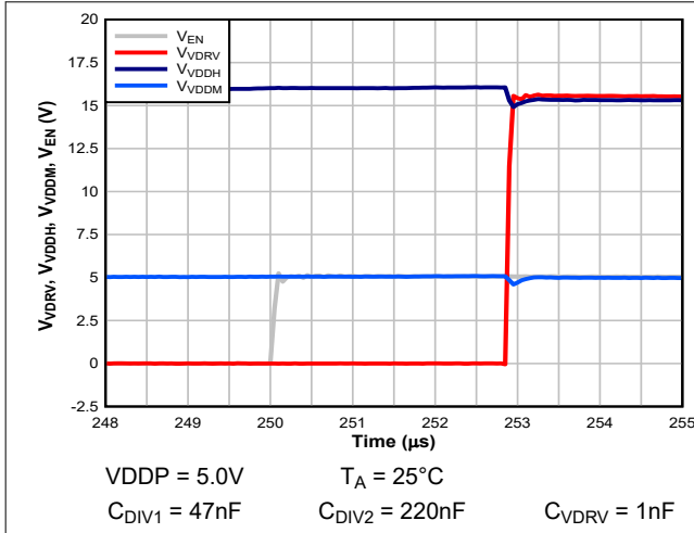
图 6-3. t LH_VDRV
