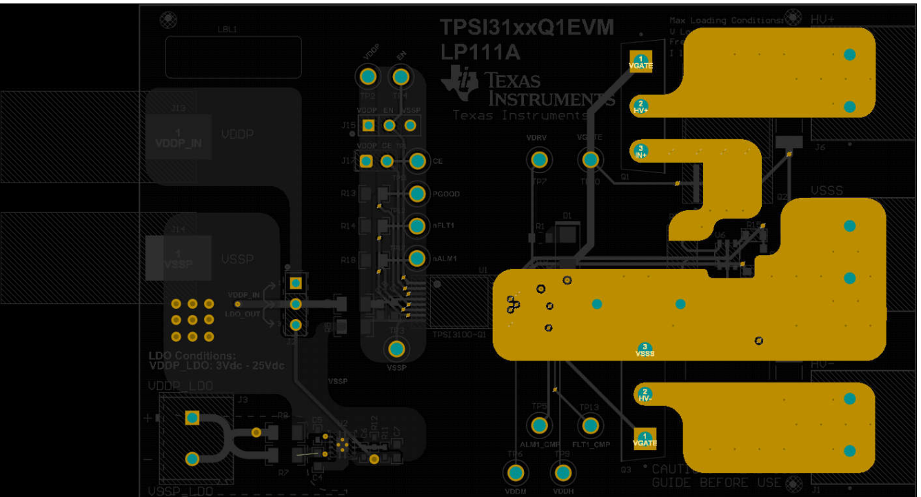
图 9-6. 信号层 1
