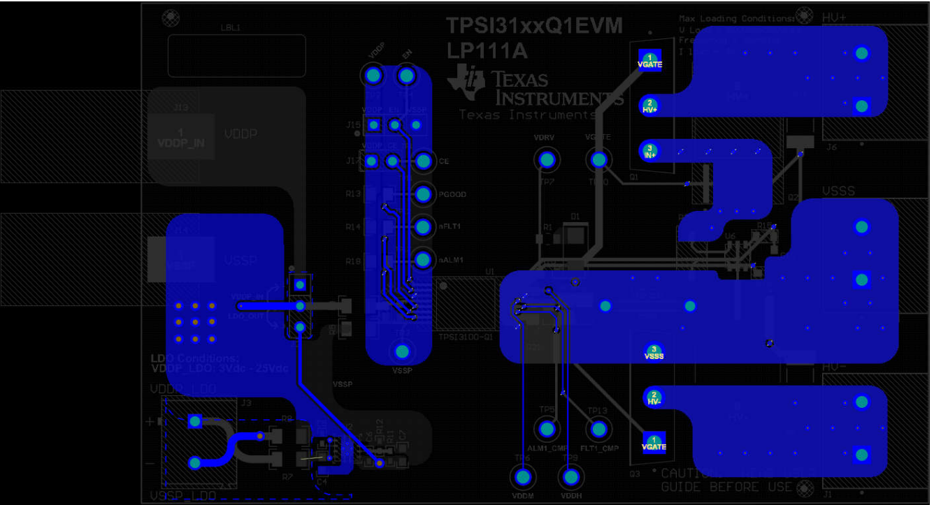
图 9-5. 底层
