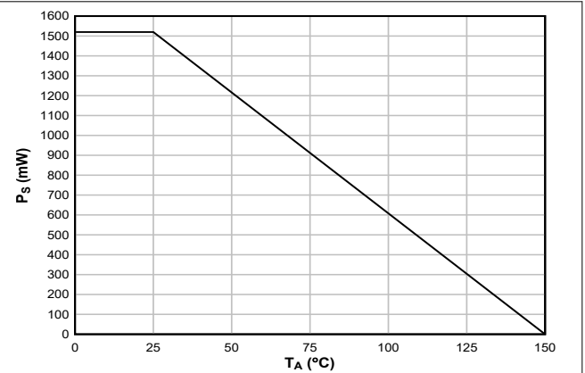
图 6-2. 根据 VDE 和 IEC 标准限制功率的热降额曲线
