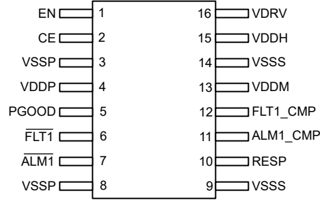
图 5-4. TPSI313x-Q1 DVX 封装，16 引脚 SSOP（顶视图）
