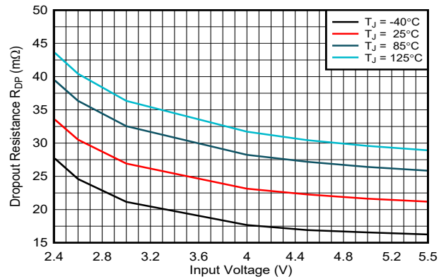
图 6-4. Dropout Resistance R DP
