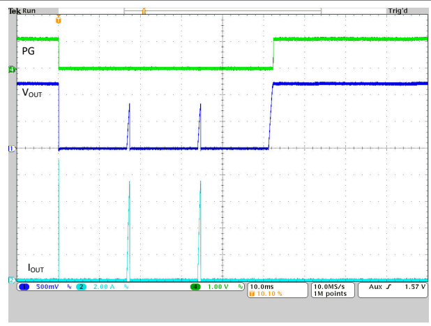
图 8-37. HICCUP Short-Circuit Protection
