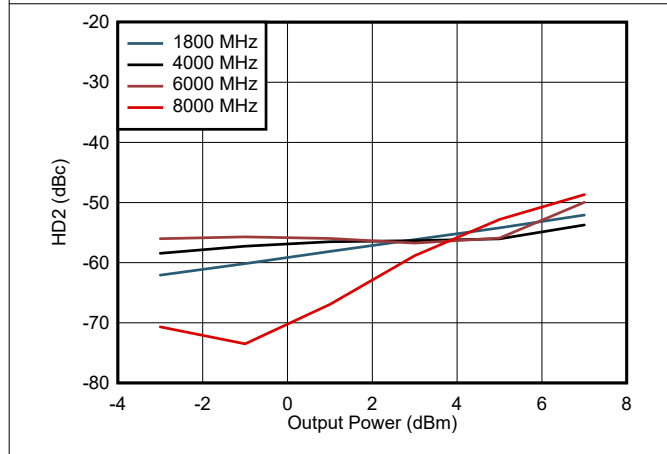
图 6-63. HD2 vs Output Power
