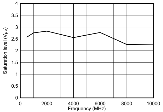
图 6-74. Saturation Voltage
