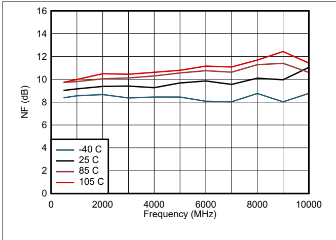
图 6-67. NF Across Temperature
