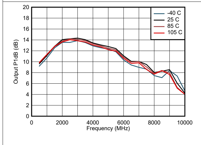
图 6-65. Output P1dB Across Temperature
