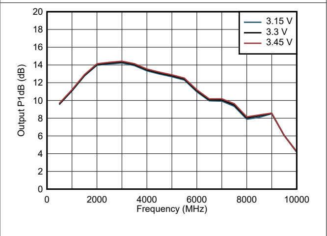
图 6-66. Output P1dB Across VDD
