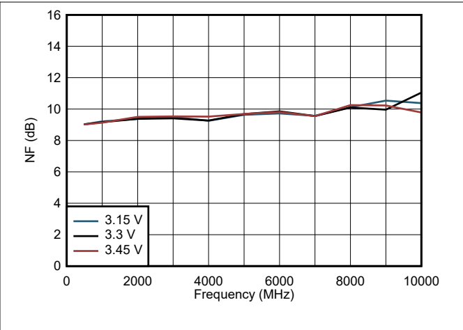
图 6-68. NF Across VDD
