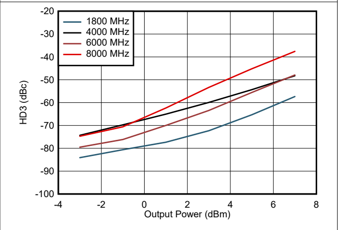
图 6-64. HD3 vs Output Power
