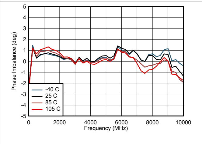
图 6-70. Phase Imbalance
