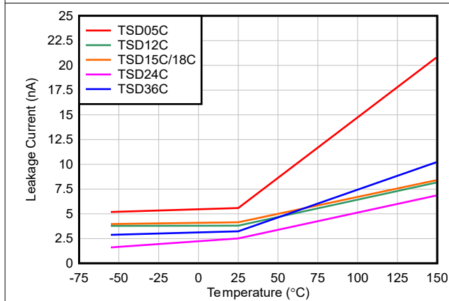
图 5-9. 漏电流与温度间的关系
