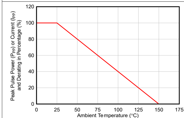
图 5-11. 峰值脉冲功率降额曲线
