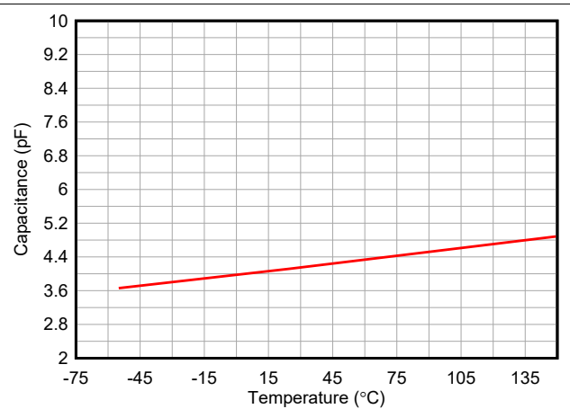
图 5-10. 电容与温度间的关系 - TSD05C
