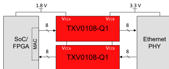
RGMII 应用中的 TXV0108-Q1
