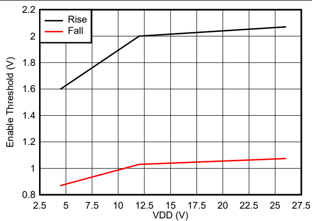
图 6-10. Enable Threshold
