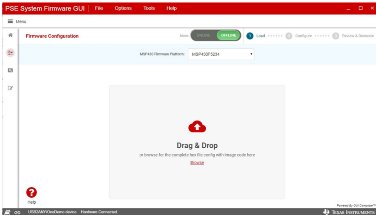
图 3. GUI Startup
