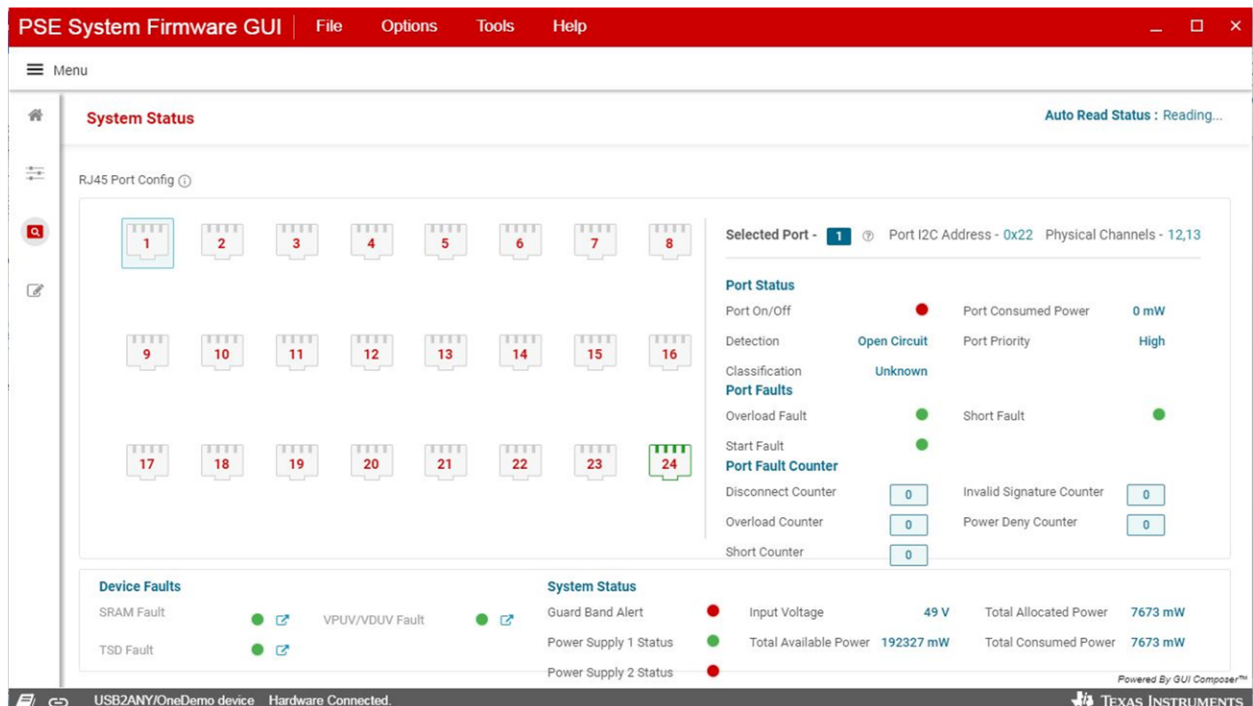
图 11. GUI Status Page
