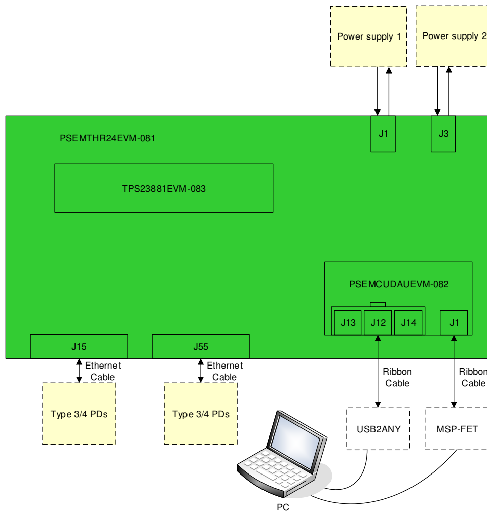
图 2. Ecosystem Setup
